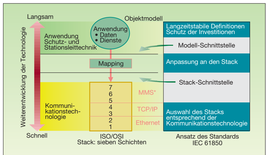
Bild 2 Schichtenansatz
